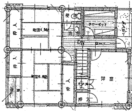
2階平面図
